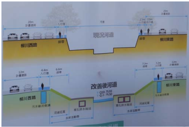
拡幅後の横断面図
